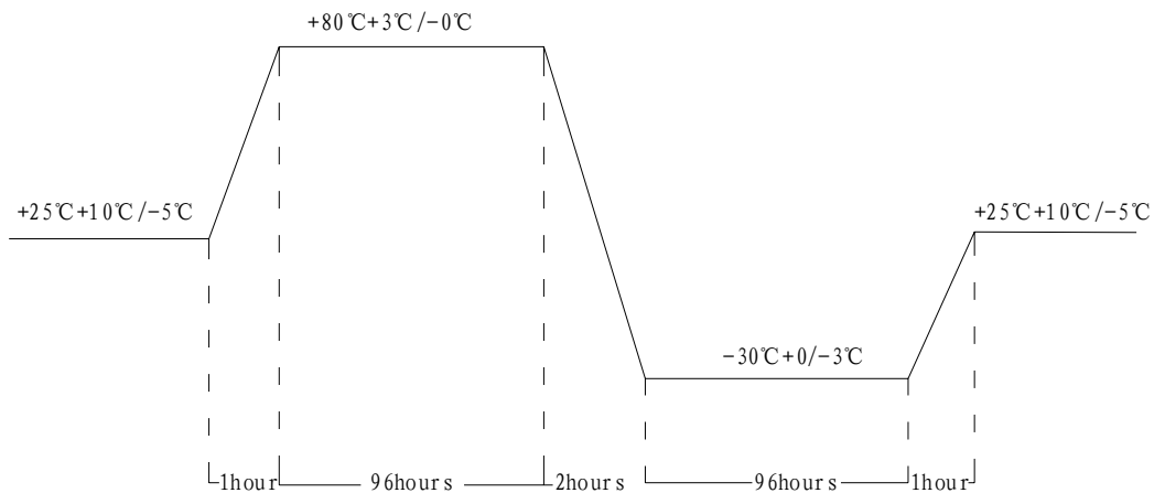
FIG1 TEMP. TEST
